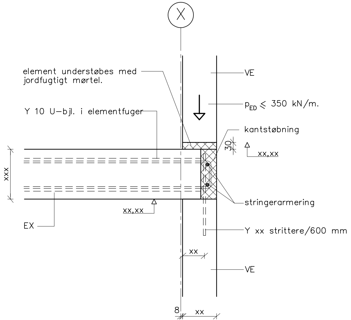
Samling mellem EX / VE (bærende) ved etagekryds.
